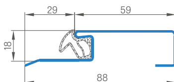
Seuil en tôle inox
