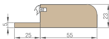
Seuil en bois dur
