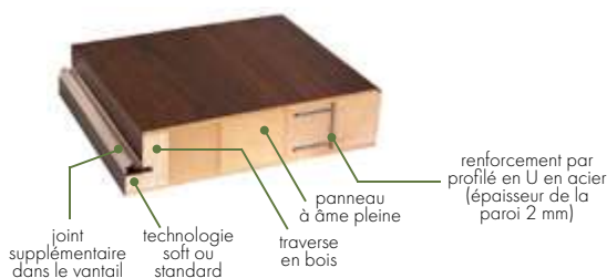
COUPE TRANSVERSALE DU VANTAIL DE PORTE HERSE 32 dB
