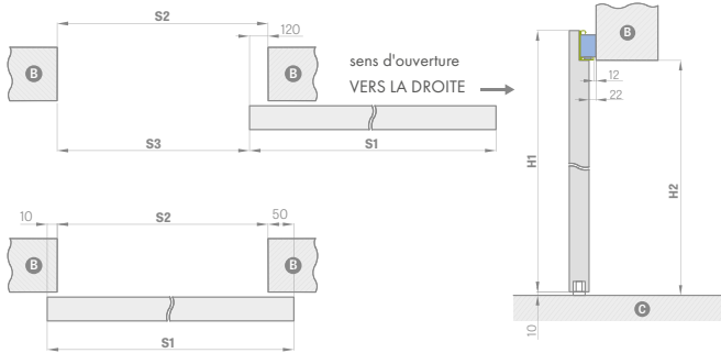
Vantail MAGIC, coloris CHÊNE PREMIUM, poignée ovale
