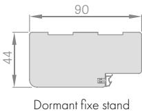
Dormant fixe stand
