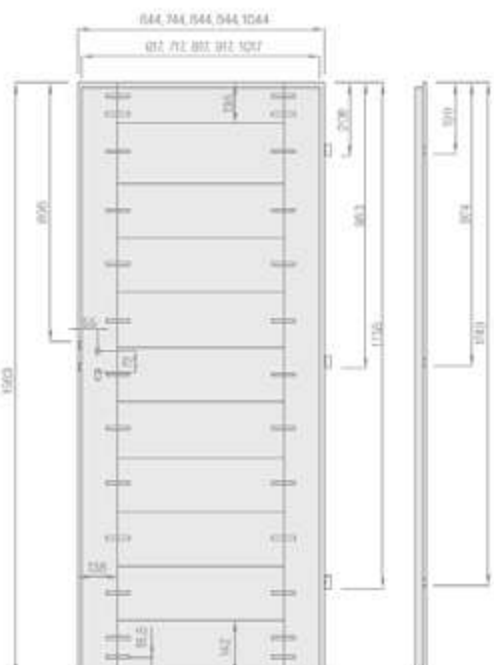
vantail avec paumelles visibles
