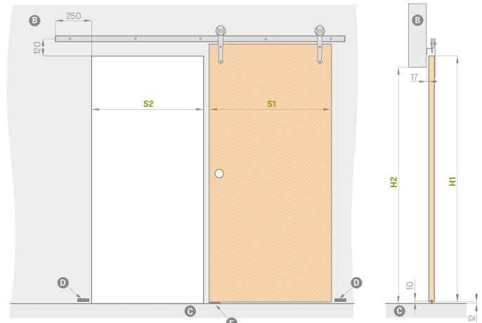
Vantail LOFT, coloris CHÊNE ST CPL, poignée ronde, support pour le vantail RETRO
