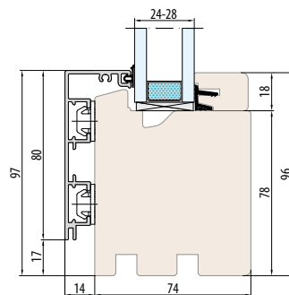
SYSTÈME ESPERIA LIFE 74 ALU-Fix
