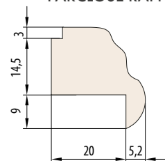
PARCLOSE RAPPORTÉE
