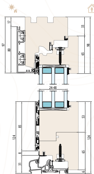
SYSTÈME ESPERIA LIFE 74 ALU portes-fenêtres à un vantail avec seuil bas
