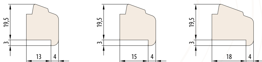
PARCLOSE RAPPORTÉE
