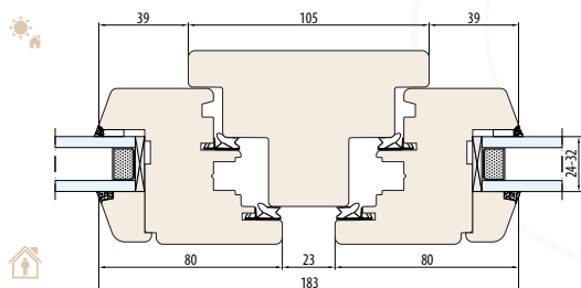
SYSTÈME NATURO 68 meneau fixe 105 mm (section horizontale)
