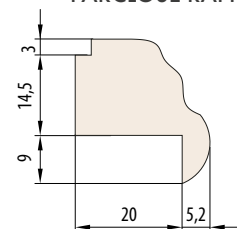
PARCLOSE RAPPORTÉE
