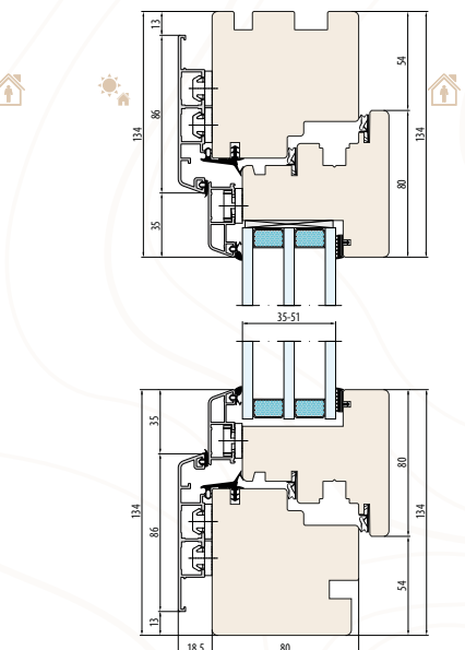
SYSTÈME NATURO 80 ALU GEMINI CLASSIC découpe pour l'appui de fenêtre intérieur
